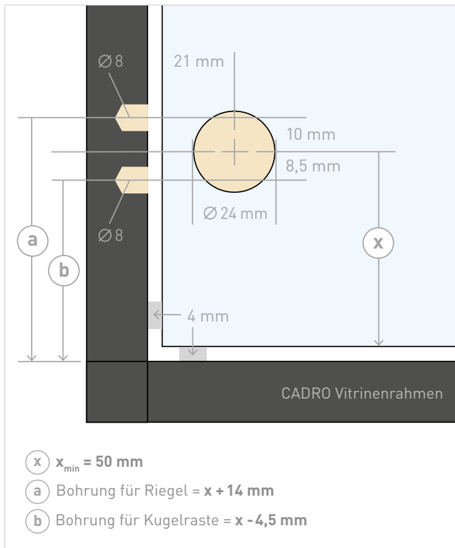
Bohrmaße für Glastür DIN rechts
