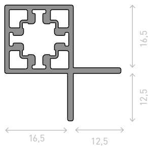
Eckprofil 9 303 886 / 9 303 911
