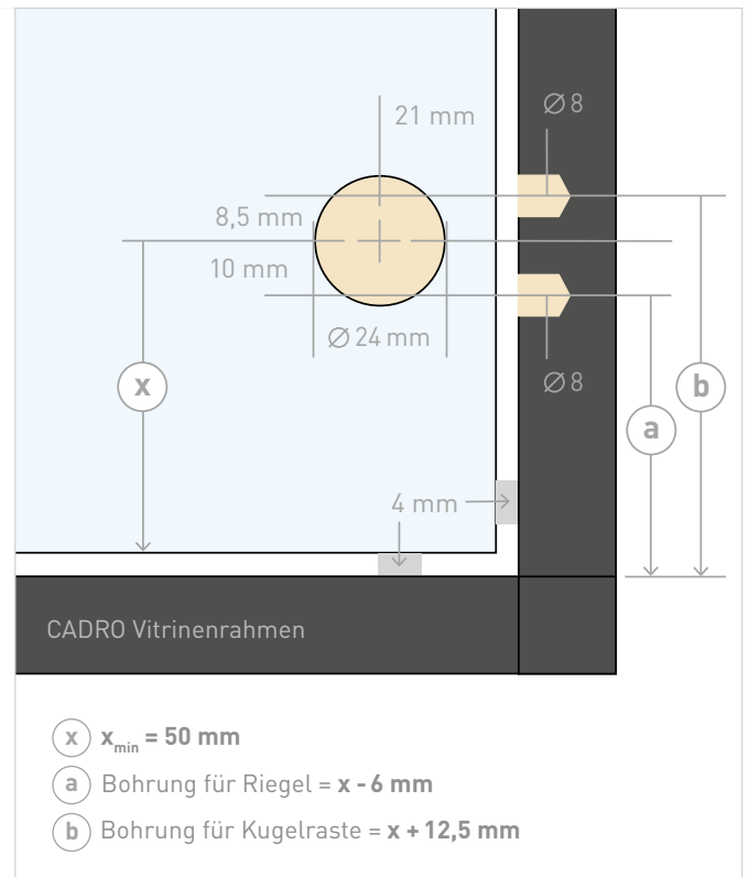
Bohrmaße für Glastür DIN links
